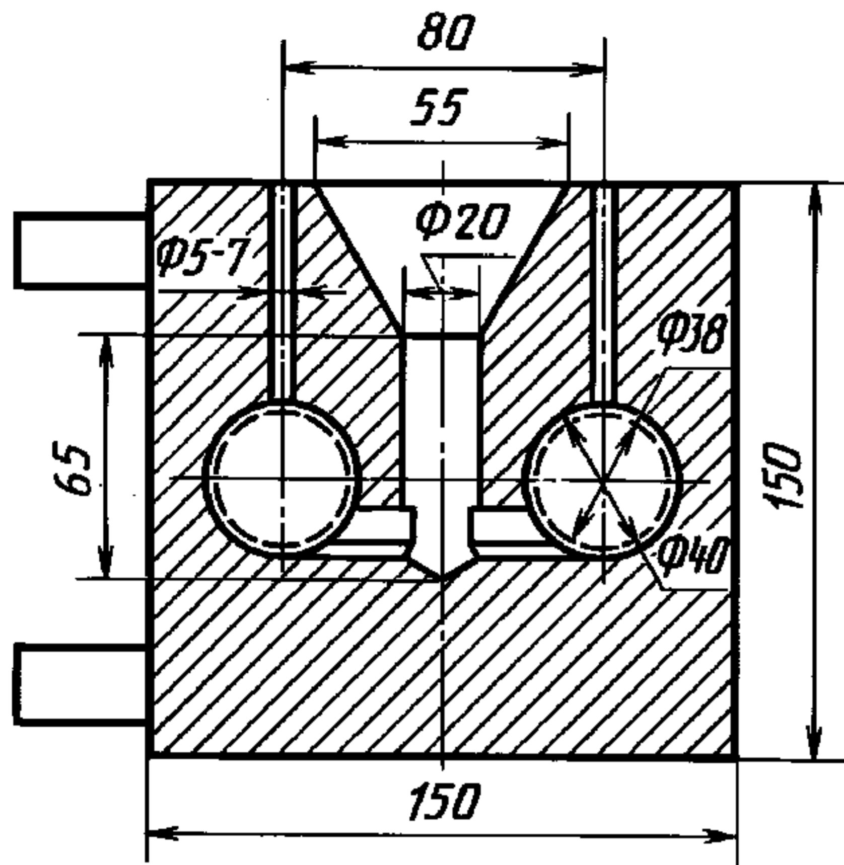
Двухдисковая изложница для отбора проб чугуна
