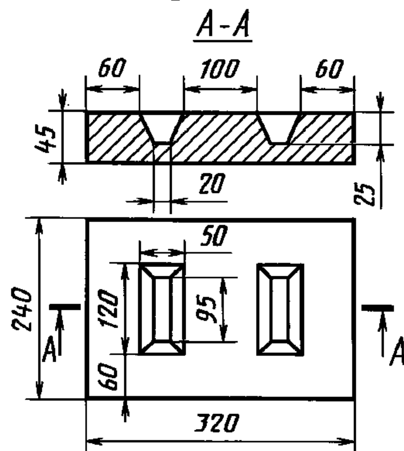
Изложница с формой призмы
