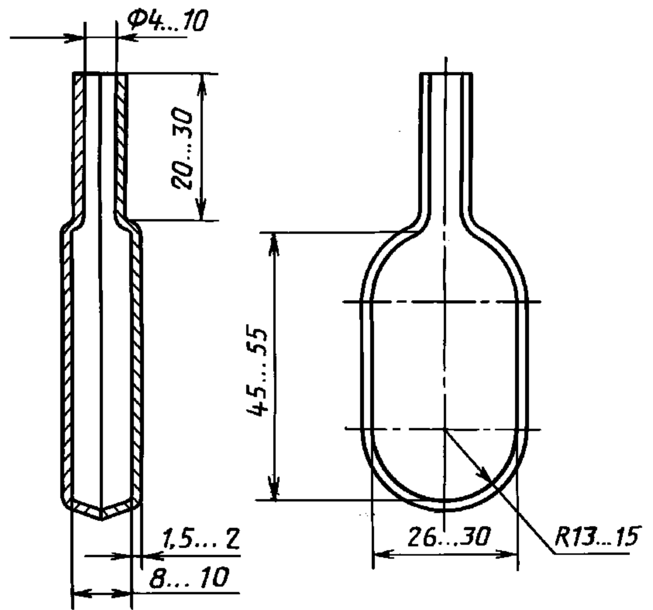
Пробница разъемная для отбора проб жидкой стали
