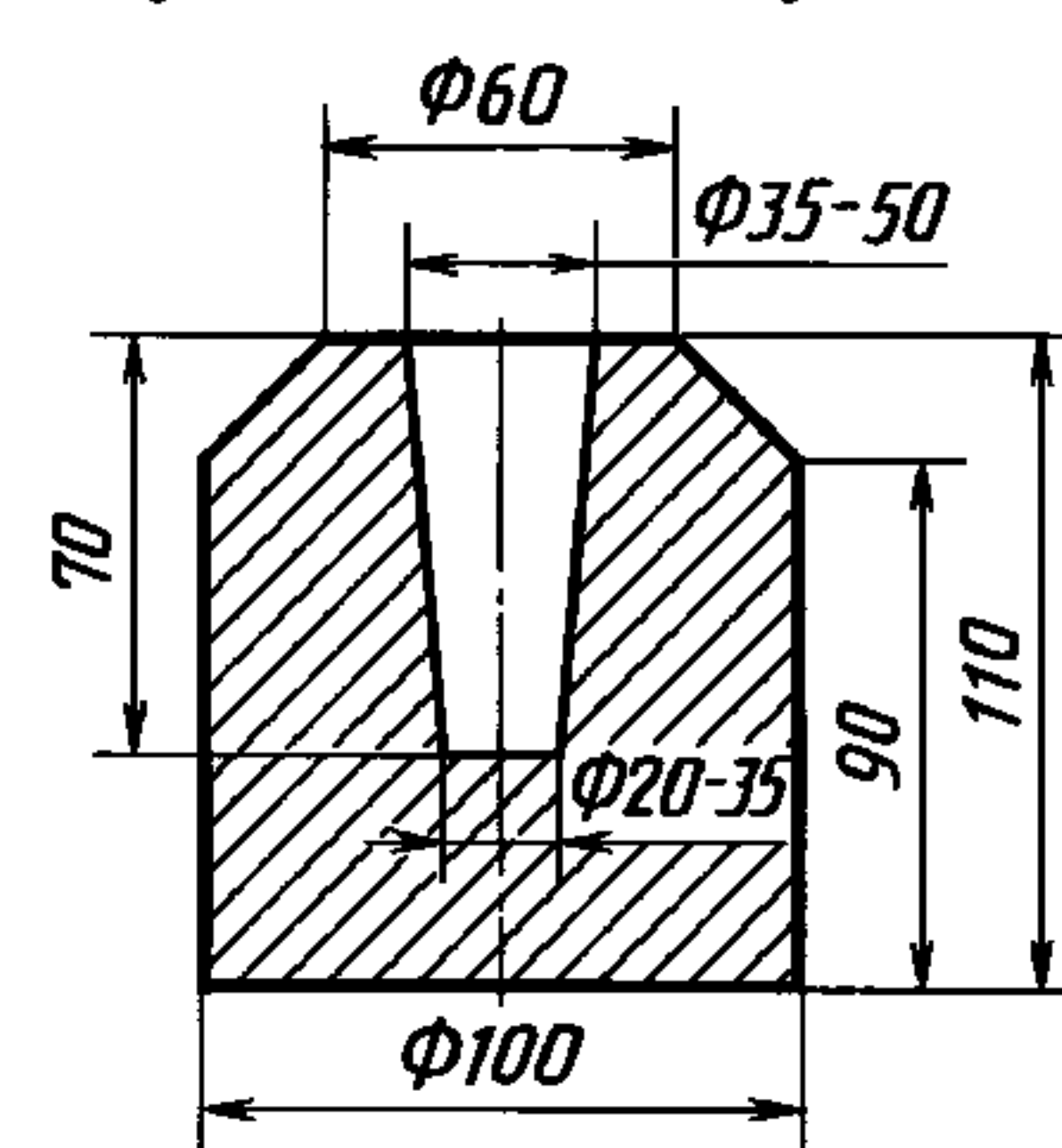
Изложница с формой усеченного конуса
