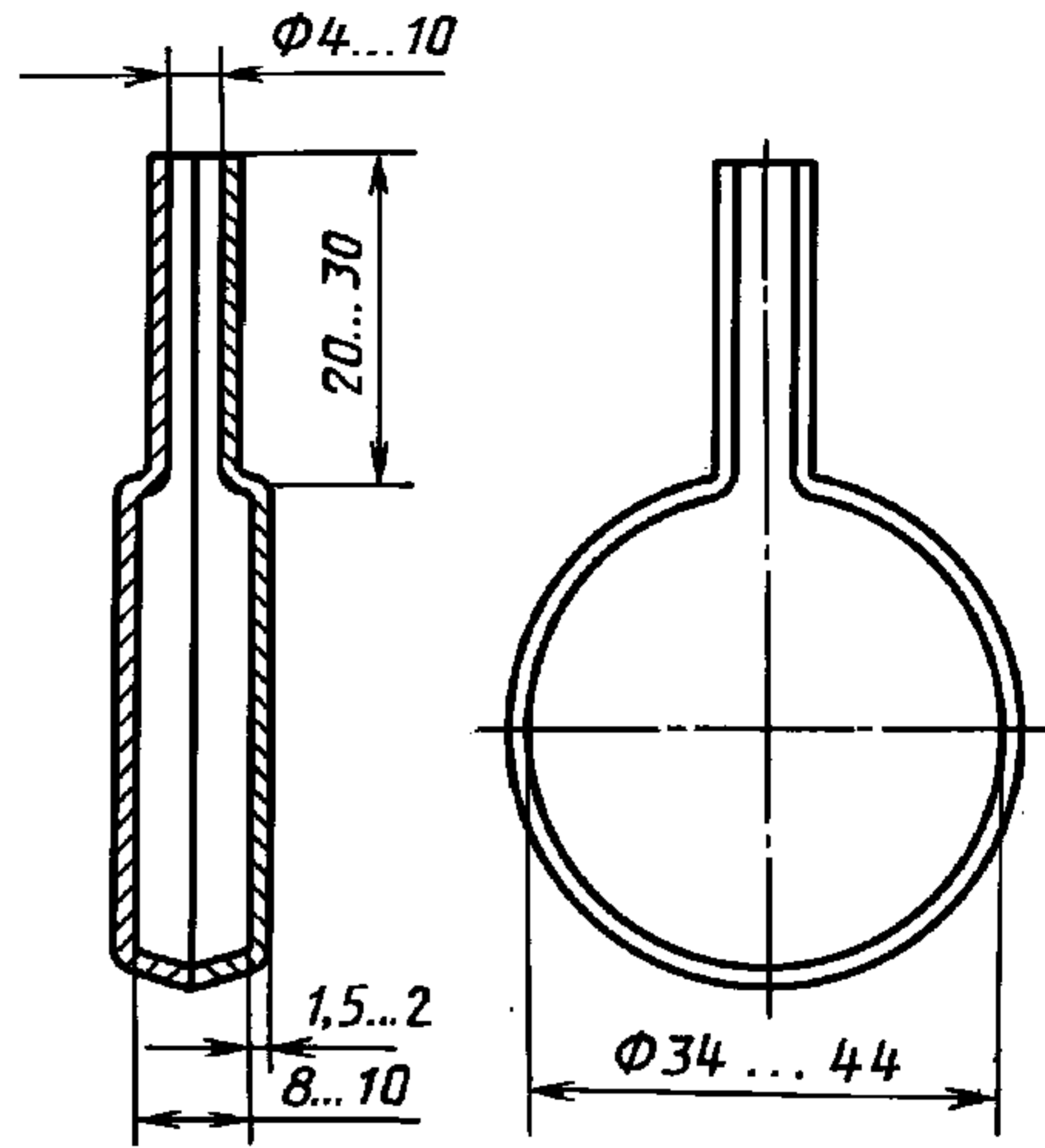
Пробница разъемная для отбора проб жидкой стали
