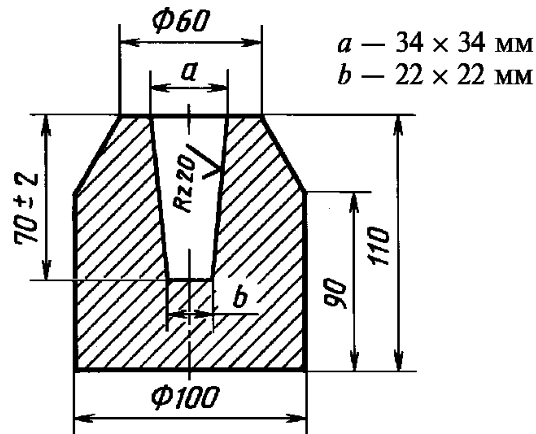
Изложница с формой усеченной четырехгранной пирамиды
