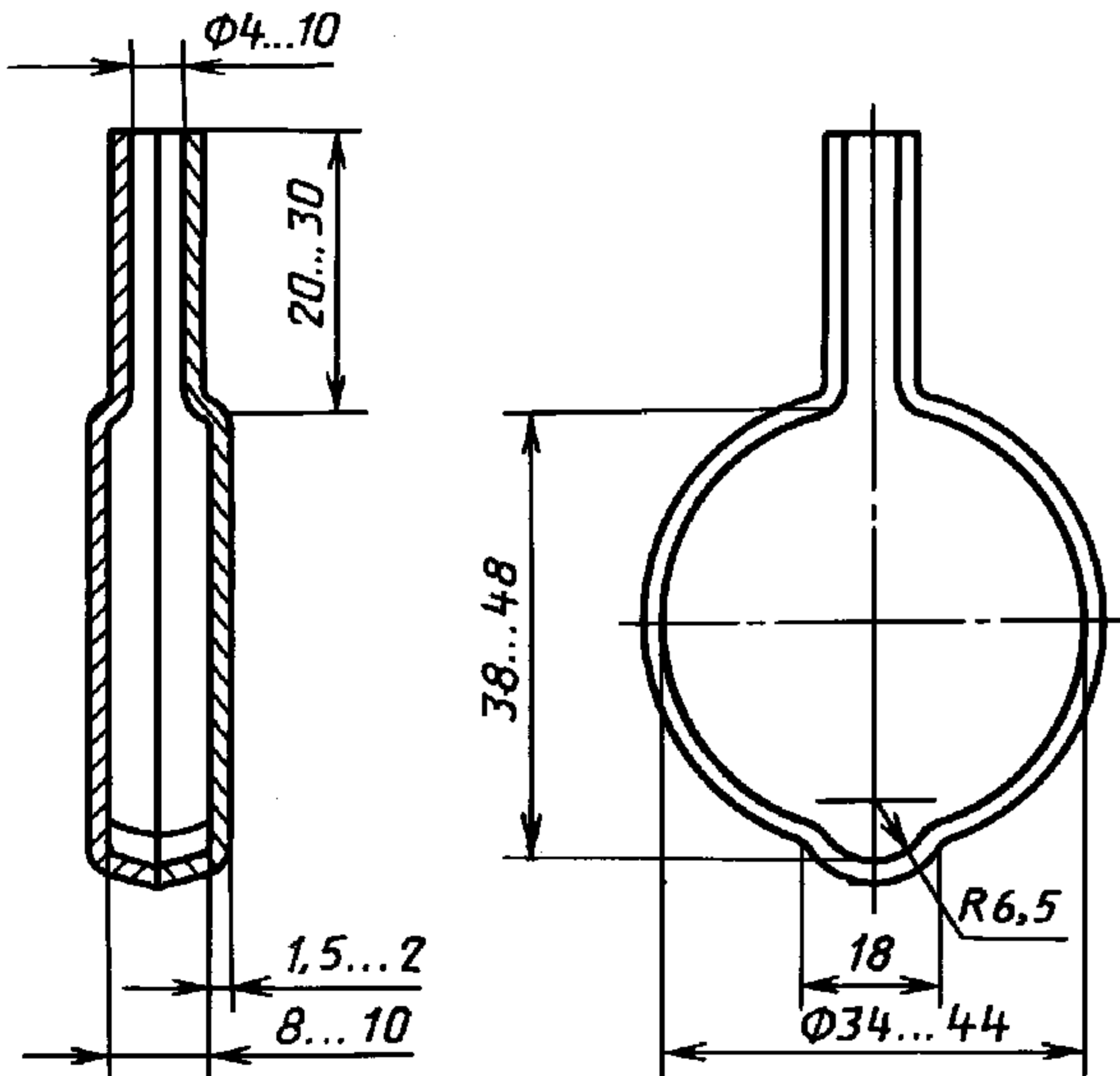
Пробница разъемная для отбора проб жидкой стали
