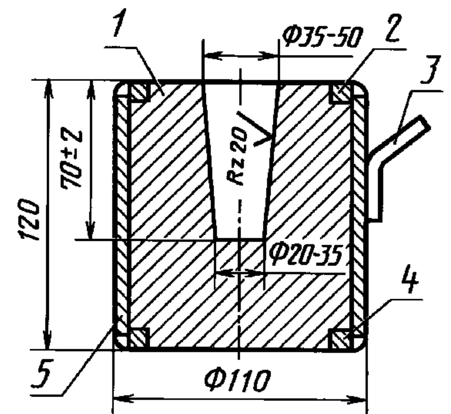
Комбинированная изложница с формой усеченного конуса
