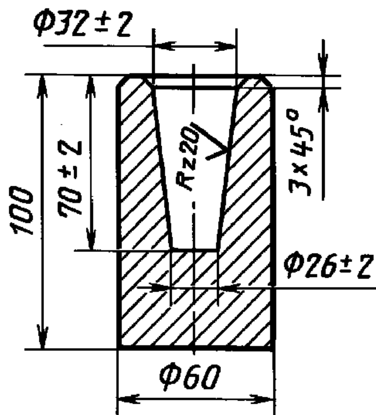
Изложница с формой усеченного конуса
